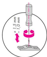
Výškové seřízení zvedavače křídla
