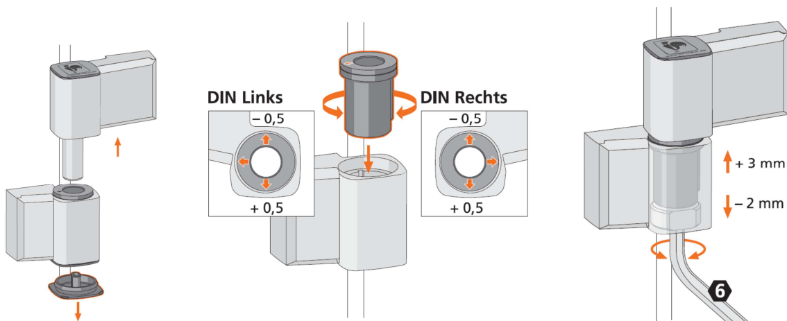
Sejmutí krytky a vysazení křídla
