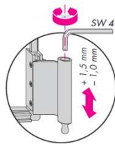
Výškové seřízení imbusovým klíčem č. 4
